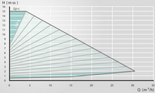
ASP 40/15 250 İNV
