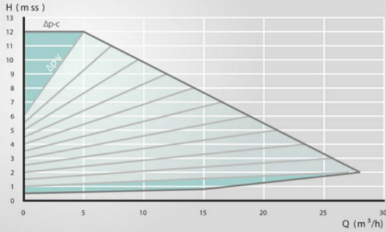
40/12 250 İNV
